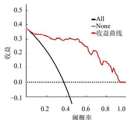
图 3 诺模图模型的决策曲线
