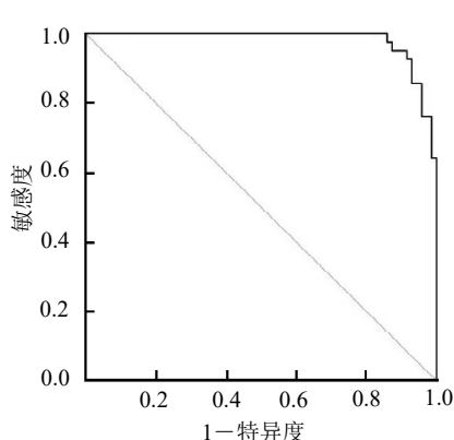
图 1 诺模图模型 ROC 曲线
